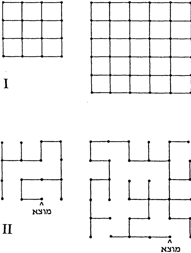
איור 2. מערכת ניקוז המבוססת על "עץ משחיל" (spanning tree) על בסיס של רשת ריבועים (על-פי Karlinger & Troutman, 1989).
