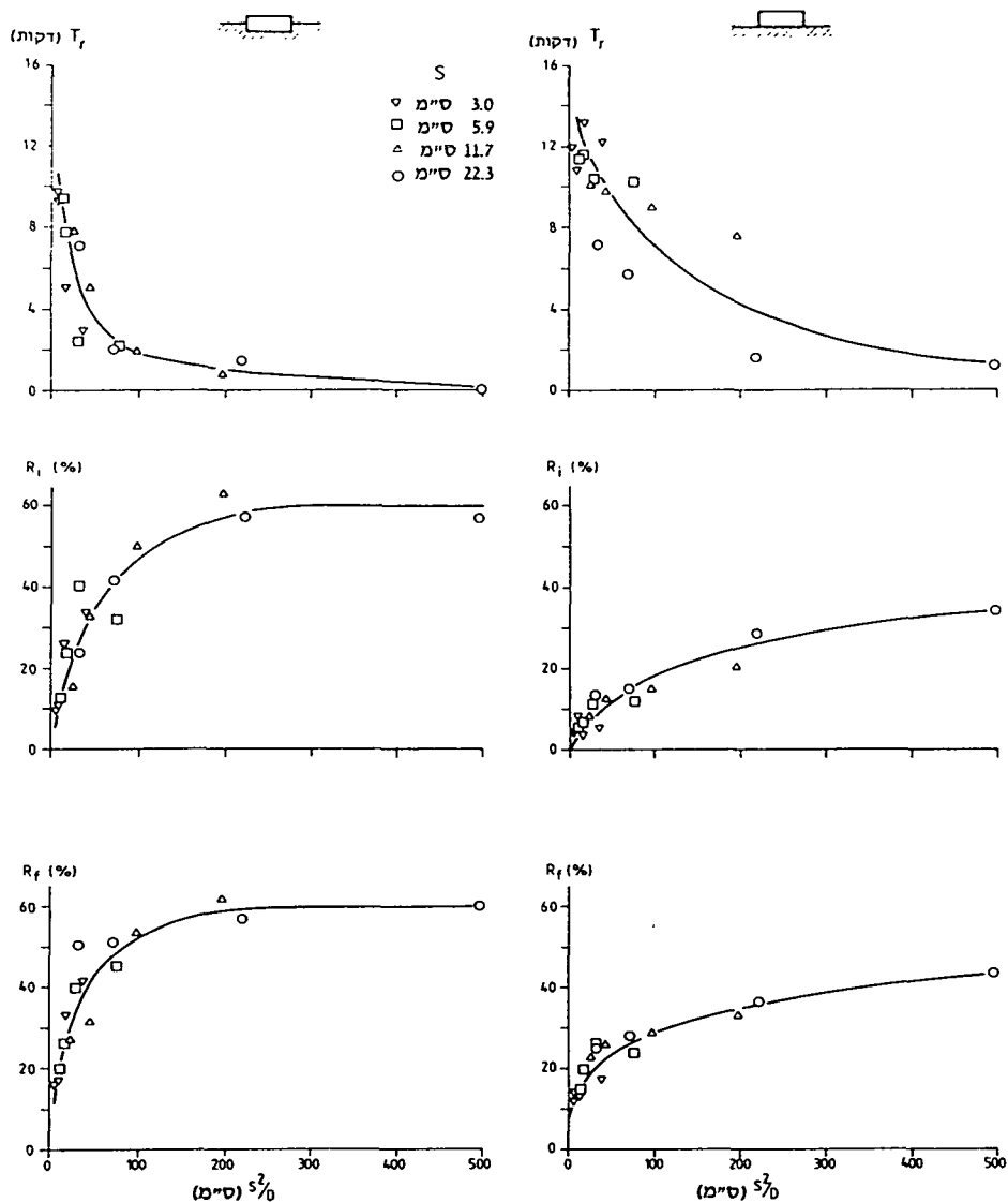
איור 8. הקשר בין R_i , R_f ו- S^2/D .
