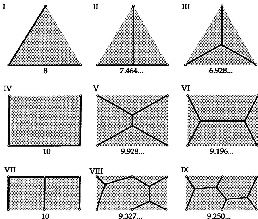
איור 3. נסיונות למציאת המרחק המינימלי המקשר 3, 4 ו-6 נקודות (על-פי Bern & Graham, 1989).
