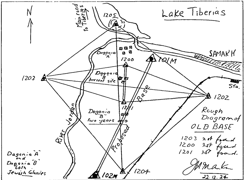
איור 3. קו הבסיס של רשת הטריאנגולציה למדידת אדמות בית-שאן
